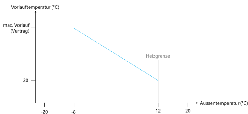
Abbildung 3: Standardheizkurve für Wärme 70 und Wärme 40
